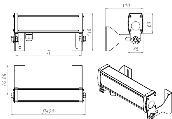
Габаритні розміри.
