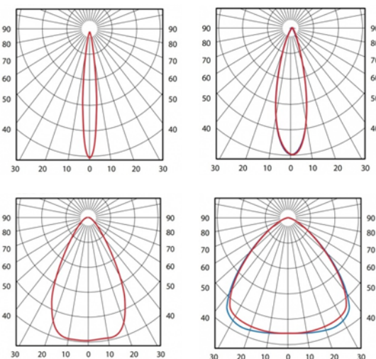
Діаграма КСС.
